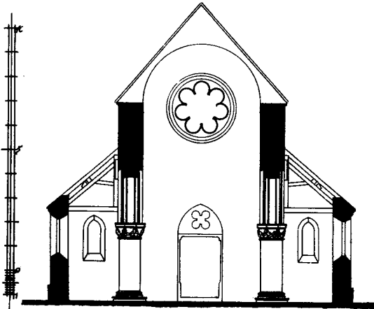
QUERSCHRITT D. D. SCHIFF
