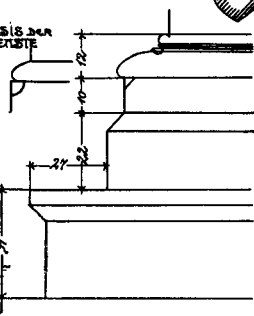
BASIS DER SCHIFFS- SÄULEN
