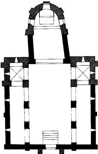
2b. Plan et vue perspective supposés de l'église au début du XII e siècle.
