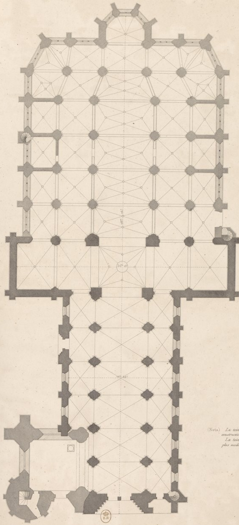
PLAN GÉNÉRAL ÉTAT ACTUEL DE L'ÉGLISE SAINT ETIENNE DE BEAUVAIS (Picardie)
